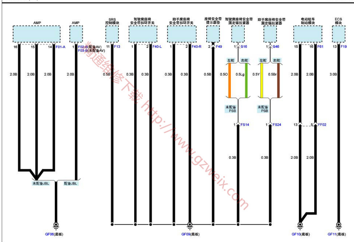
搭铁分布(17)
